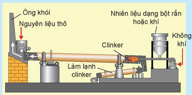
Hình 5.6. Sơ đồ dây chuyền sản xuất clinker
