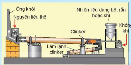
Hình 5.6. Sơ đồ dây chuyền sản xuất clinker xi măng
