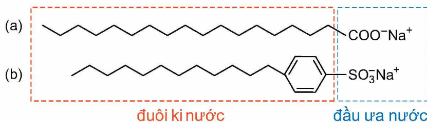
Hình 2.2. Công thức cấu tạo của một số chất hoạt động bề mặt: xà phòng (a) và chất giặt rửa phổ biến (b)
